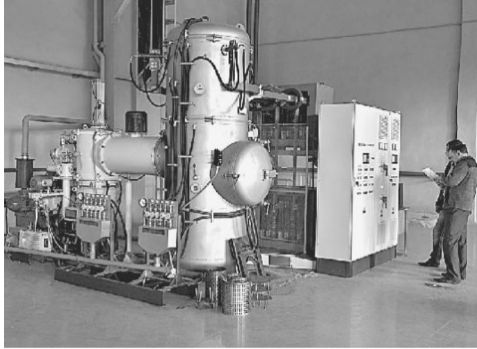
НА УЧАСТКЕ ВАКУУМНЫХ ПЕЧЕЙ. Здесь установлено самое современное оборудование.
